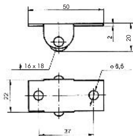
KÓŁKO K003
