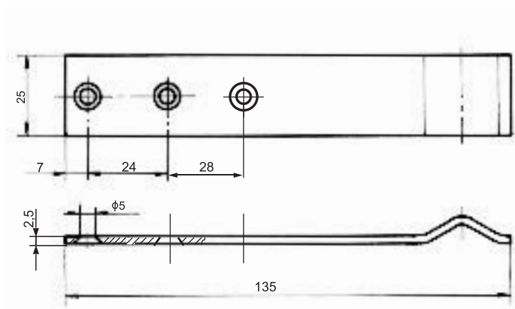
NAJAZD N002
