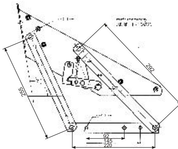
PODNOŚNIK WERSALKI BEZKŁOCKOWY 002.01.MA
