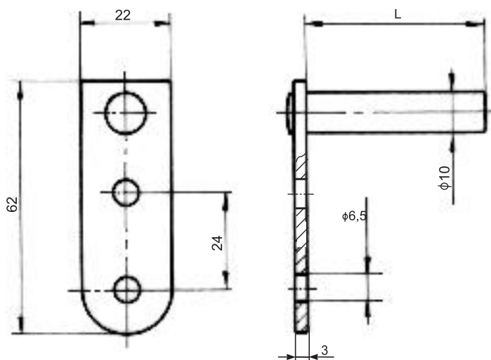
KORBKA 3+2+1
