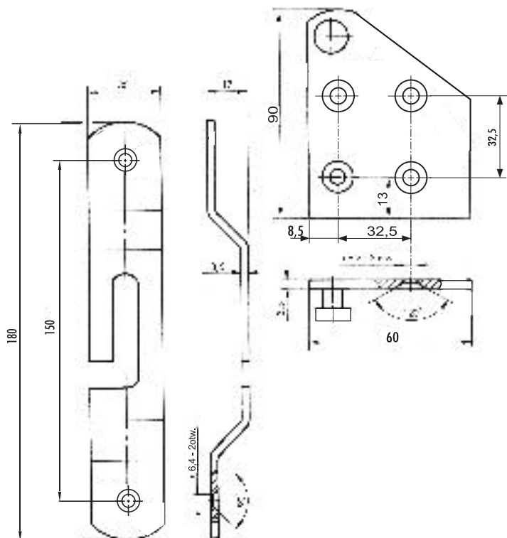
ZAWIAS "AMERYKANKI" 007.04.OC
