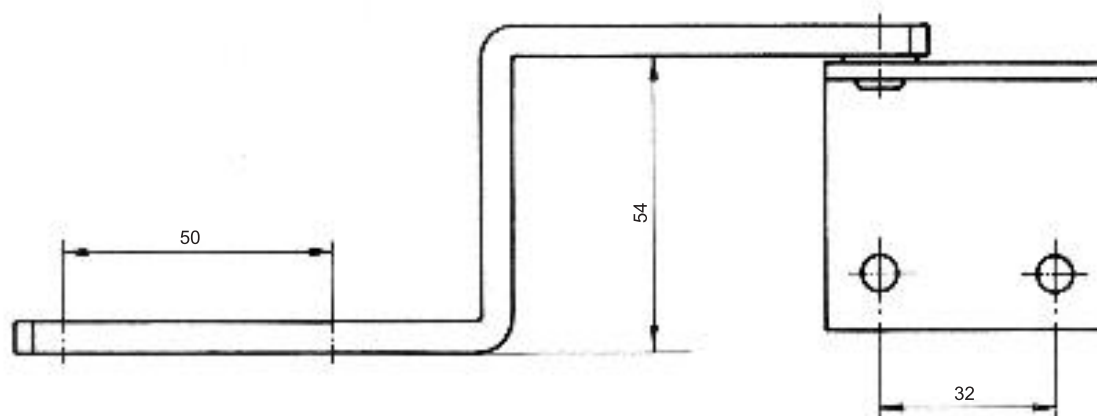
ŚMIGI DUŻE Z021
