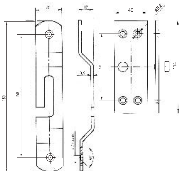
ZAWIAS "AMERYKANKI" 007.05.OC
