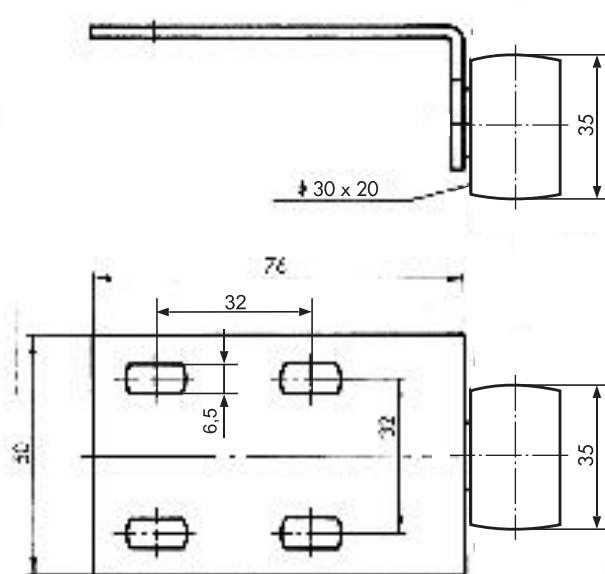
BLASZKA KĄTOWA Z KÓŁKIEM B008
