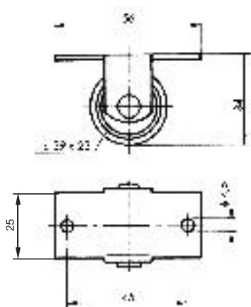
KÓŁKO K010
