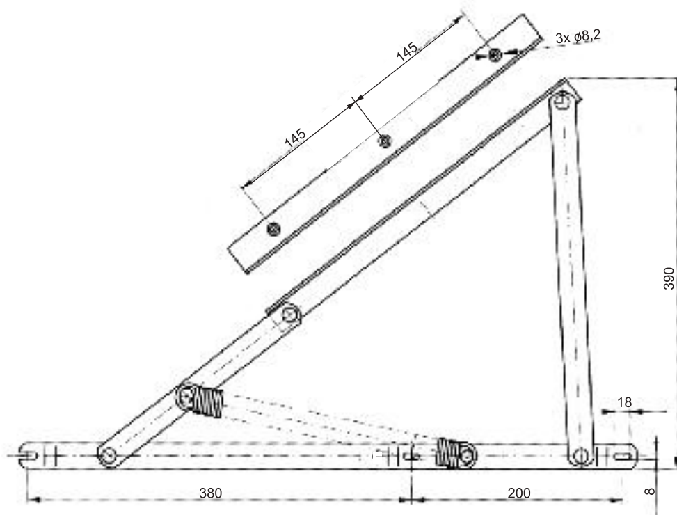
PODNOŚNIK TAPCZANOWY NAROŻNIKA 015.01.MA / OC
