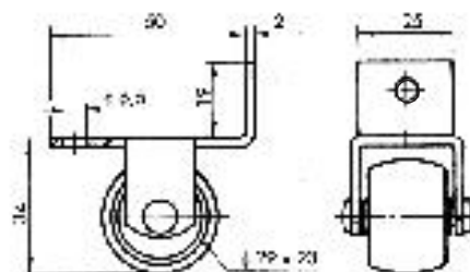
KÓŁKO K009
