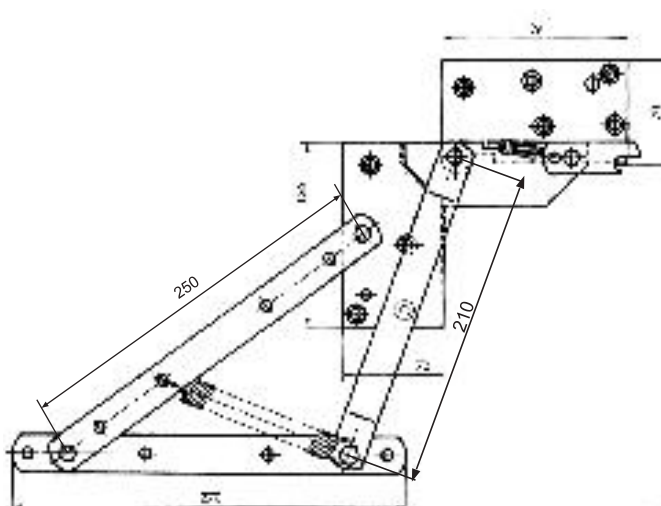
PODNOŚNIK WERSALKI KŁOCKOWY 003.01.MA
