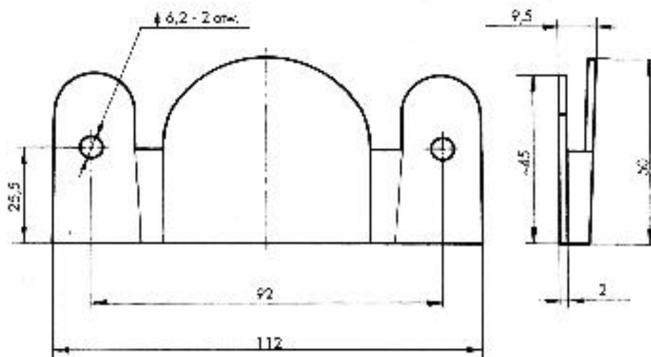
ZŁĄCZE BOKÓW Z010
