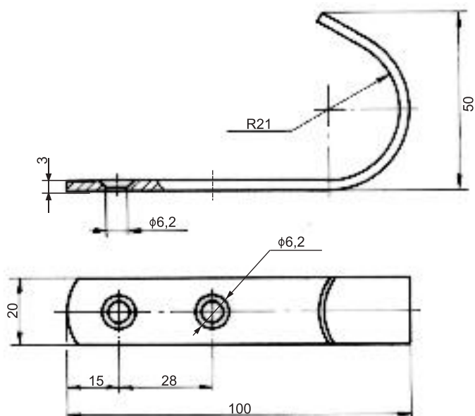
HACZYK H003
