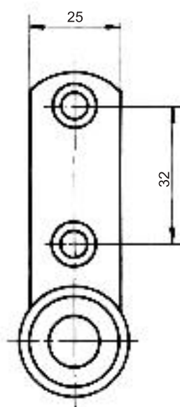
BLASZKA Z KÓŁKIEM B012
