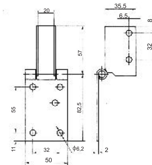
ZAWIAS Z003
