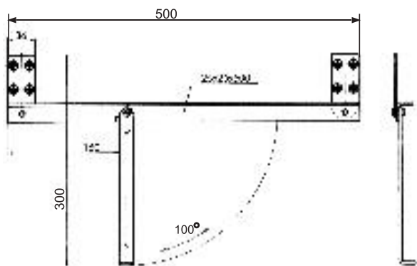
PODNOŚNIK "AMERYKANKI" 007.01.MA
