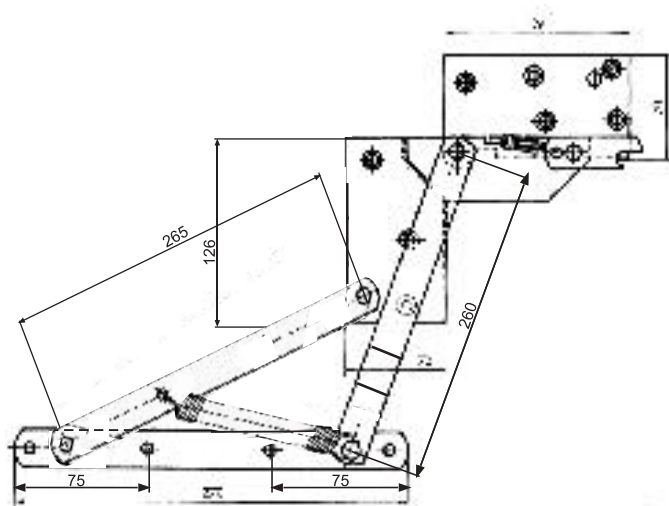
PODNOŚNIK WERSALKI KŁOCKOWY II 003.02.MA
