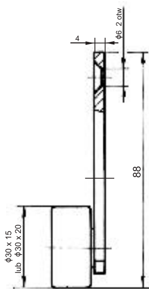
BLASZKA Z KÓŁKIEM B012
