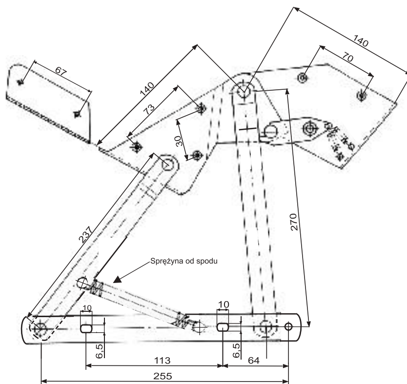
PODNOŚNIK GALAKSIA WEWNĘTRZNA 004.02.OC
