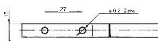
HACZYK H002
