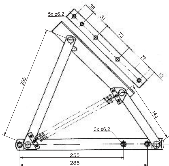
PODNOŚNIK TAPCZANOWY DUŻY 014.01.MA / OC
