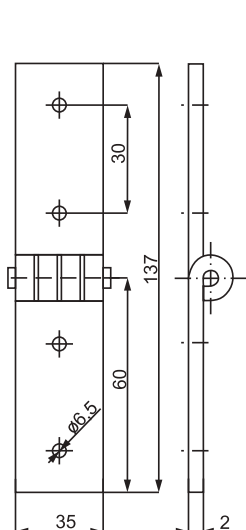
ZAWIAS Z006
