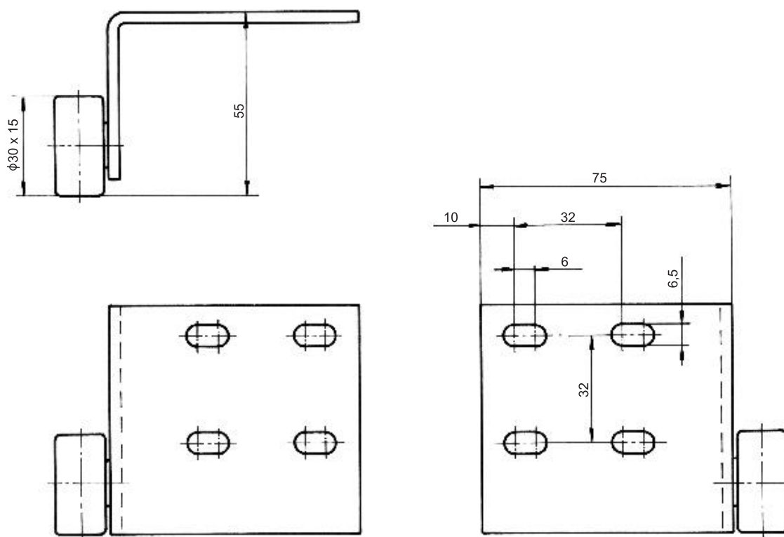
BLASZKA Z KÓŁKIEM B006 (PRAWĘ, LEWE)
