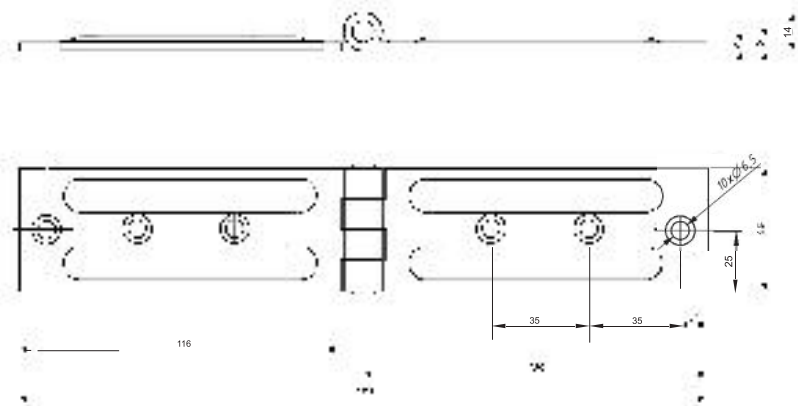
ZAWIAS Z005
