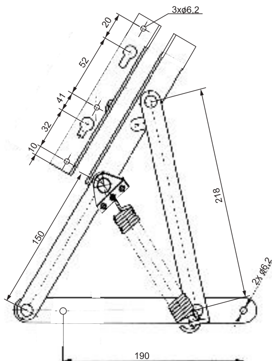
PODNOŚNIK TAPCZANOWY ŚREDNI 013.01.MA / OC
