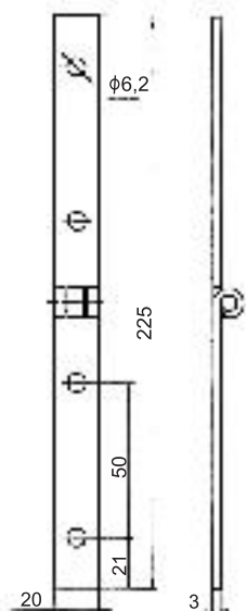
ZAWIAS Z004
