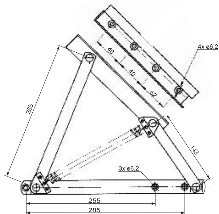
PODNOŚNIK TAPCZANOWY DUŻY Z WSUWKĄ 014.02.MA / OC
