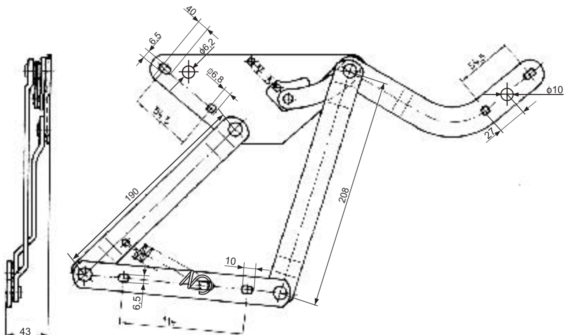
PODNOŚNIK CARO ODWROTNY - WEWNĘTRZNY 005.02.OC
