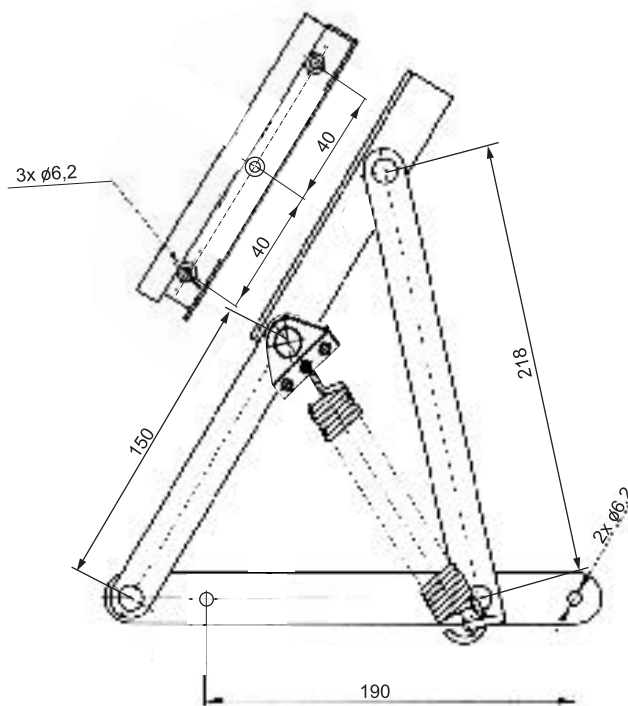
PODNOŚNIK TAPCZANOWY ŚREDNI Z WSUWKĄ 013.02.MA / OC
