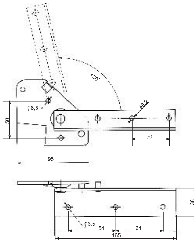
PODNOŚNIK ZAGŁÓWKA II 010.02.OC
