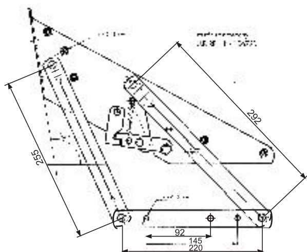
PODNOŚNIK WERSALKI BEZKŁOCKOWY WEWNĘTRZNY 002.02.MA
