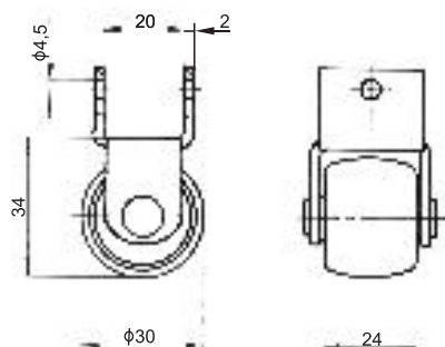
KÓŁKO K007
