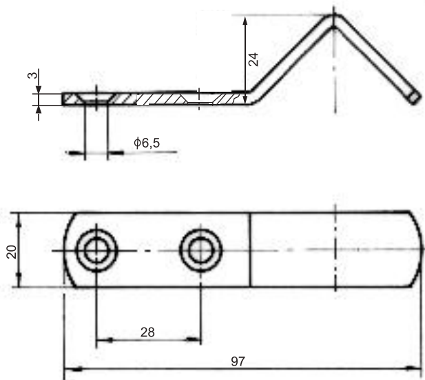
HACZYK H011
