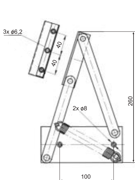
PODNOŚNIK TAPCZANOWY Z WSUWKĄ 012.02.MA
