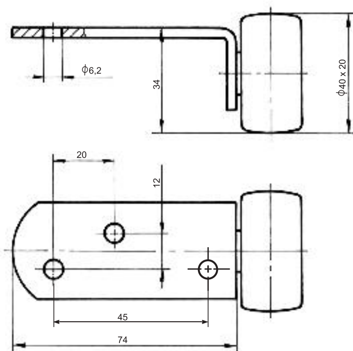
BLASZKA Z KÓŁKIEM B027
