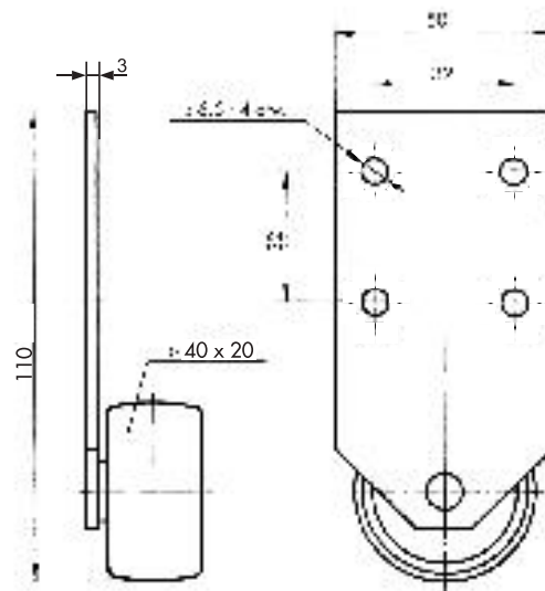
BLASZKA Z KÓŁKIEM B002
