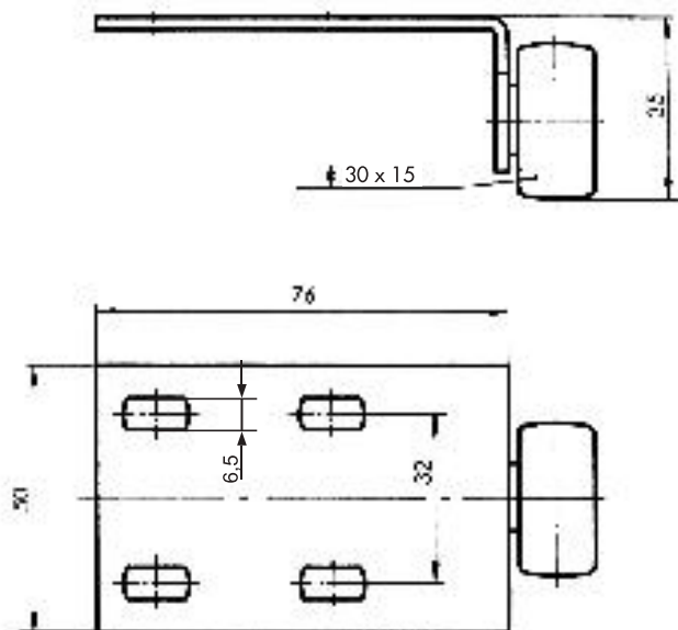
BLASZKA KĄTOWA Z KÓŁKIEM B007
