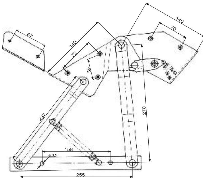
PODNOŚNIK GALAKSIA 004.01.OC
