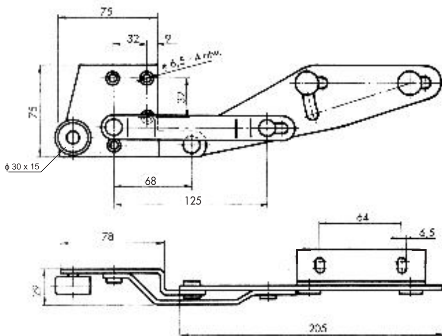
ZESTAW OKUĆ 3-2-1 Z DUŻĄ OBROTNICĄ R001
