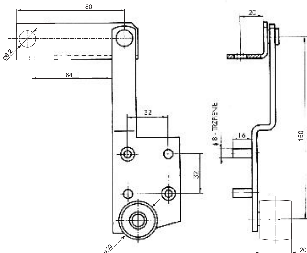
ZESTAW OKUĆ UPROSZCZONYCH 3-2-1 Z MAŁĄ OBROTNICĄ R002
