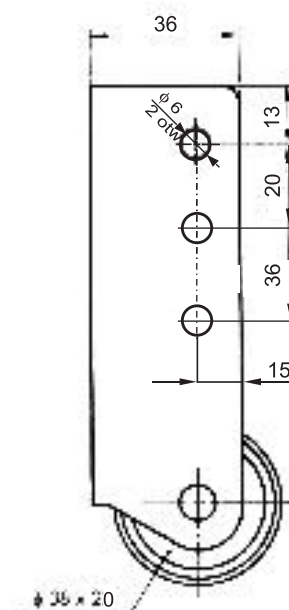
KORYTKO K025
