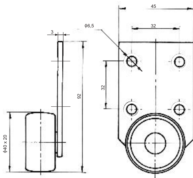
BLASZKA Z KÓŁKIEM B005
