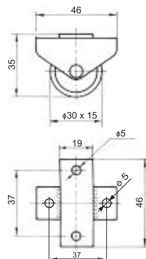
KÓŁKO K012
