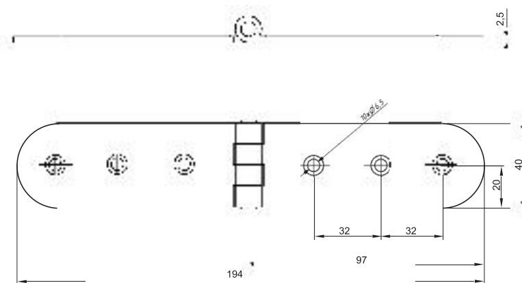
ZAWIAS Z017
