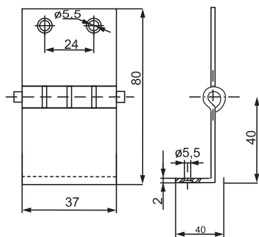
ZAWIAS Z002
