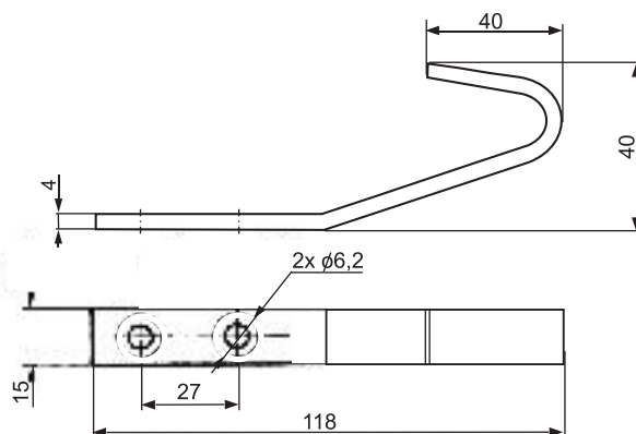
HACZYK H001
