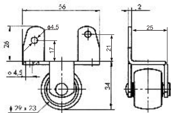
KÓŁKO K005
