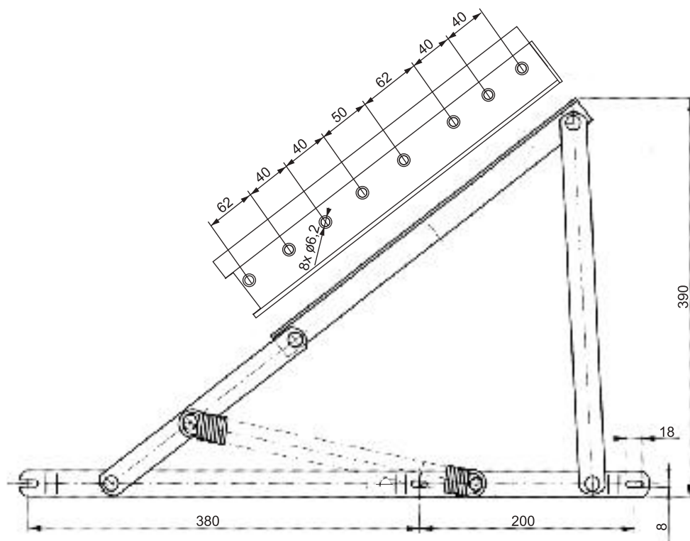
PODNOŚNIK TAPCZANOWY NAROŻNIKA Z WSUWKĄ 015.02.MA / OC
