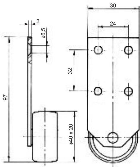
BLASZKA Z KÓŁKIEM B000
