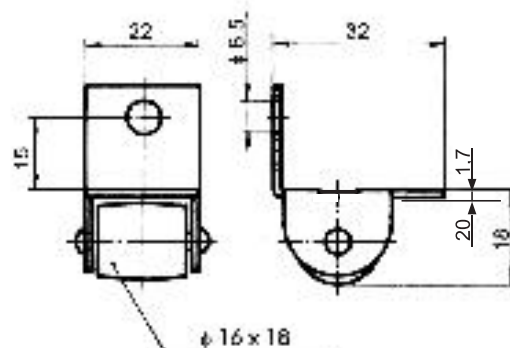
KÓŁKO K002
