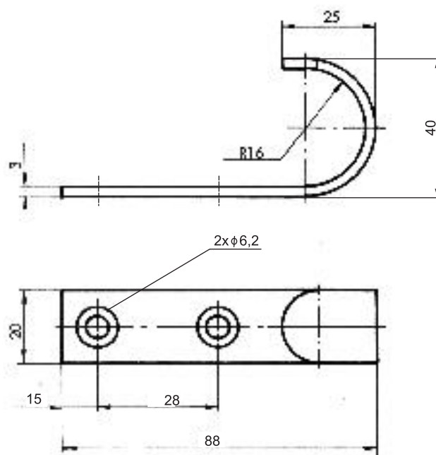
HACZYK H004
