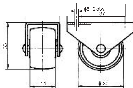
KÓŁKO K002
