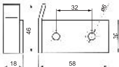
HACZYK H017
