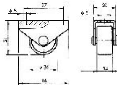
KÓŁKO K008
