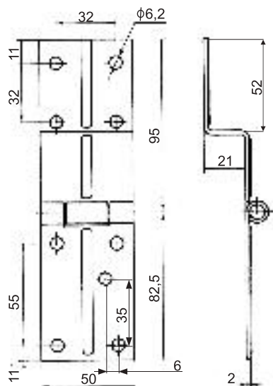
ZAWIAS Z001
