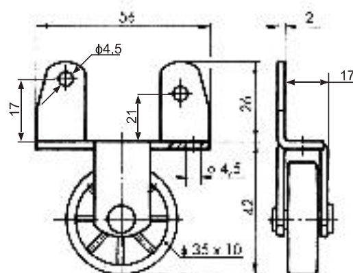
KÓŁKO K006
